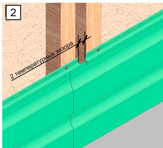
Рис. 23 Стыковка панелей горизонтального сайдинга Döcke внахлест.
