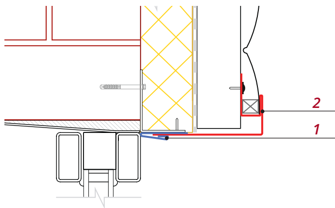
Рис. Верхний откос с Финишной планкой 48x25
